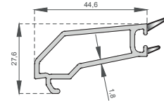
6mm.Cama Göre Çıta Glazing With 6mm.Gap A-1004
