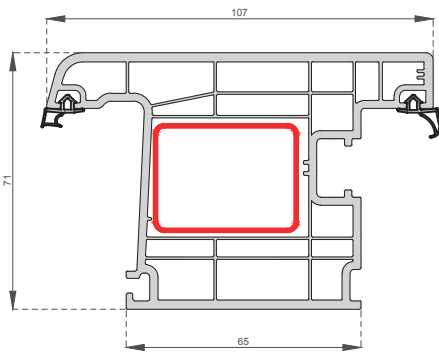
Dışa Açılır Kapı Profili Outward Opening Door C-7007
