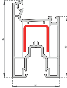
Kanat Profili Sash Profile CS-1002
