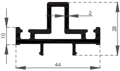
Alın Alına Kanat Kapama Alüminyum Profili Sash Lock Adapter Profile ER 7254 0,743 Kg/m
