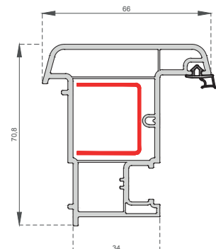
Hareketli Orta Kayıt Profili Movable Mullion Profile A-1008
