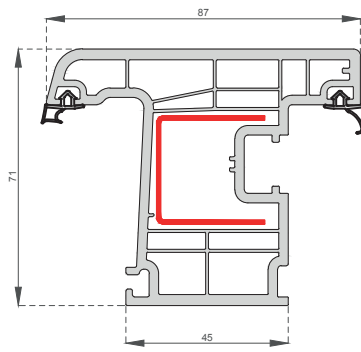
Dışa Açılır Kanat Profili Outward Opening Sash Profile C-7008
