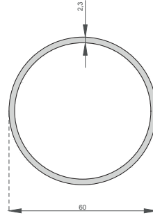
60'lık Boru Profili 60' Pipe Profile A-1014
