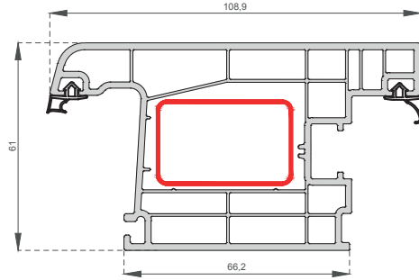
Dışa Açılır Kapı Profili Outward Opening Door C-6005
