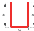
Orta Kayıt Profili Destek Sacı Mullion Profile Reinforcement Steel
