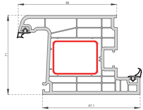
Kapı Profili Door Profile C-7106
