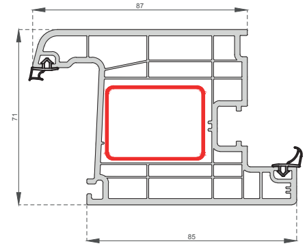
Kapı Profili Door Profile C-7006
