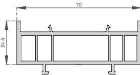
70'lik Kasa Yükseltme Profili Frame Lifting Profile A-1017
