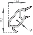
30mm.Cama Göre Çıta Glazing With 30mm.Gap A-1001
