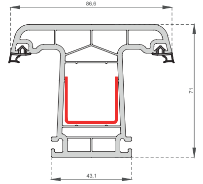
Orta Kayıt Profili Mullion Profile C-7103
