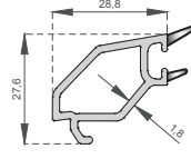
20mm.Cama Göre Çıta Glazing With 20mm.Gap A-1003
