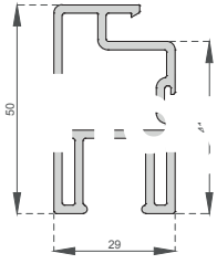
Sineklikli Kanat Profili Flyscreen Sash Profile CS-1008
