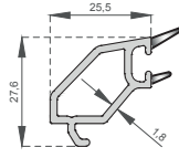
24mm.Cama Göre Çıta Glazing With 24mm.Gap A-1002
