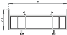
70'lik Kasa Yükseltme Profili Frame Lifting Profile A-1017
