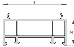
60'lık Kasa Yükseltme Profili Frame Lifting Profile A-1018
