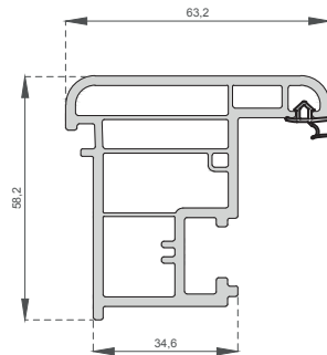
Hareketli Orta Kayıt Profili Movable Mullion Profile A-1009
