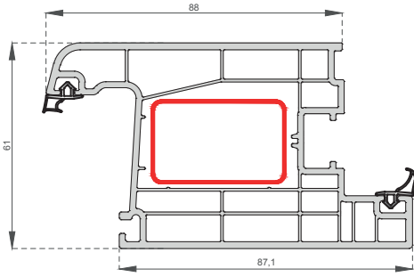
Kapı Profili Door Profile C-6004
