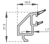
20mm.Cama Göre Çıta Glazing With 20mm.Gap A-1006
