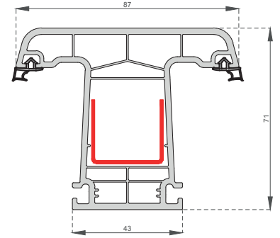
Orta Kayıt Profili Mullion Profile C-7003
