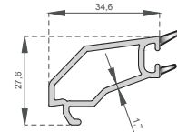
4mm.Cama Göre Çıta Glazing With 4mm.Gap A-1007
