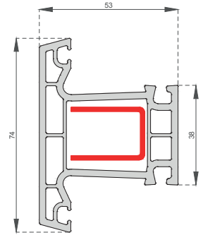
Orta Kayıt Profili Mullion Profile CS-1003
