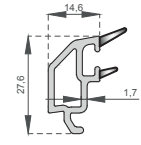
24mm.Cama Göre Çıta Glazing With 24mm.Gap A-1005
