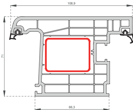
Dışa Açılır Kapı Profili Outward Opening Door C-7107
