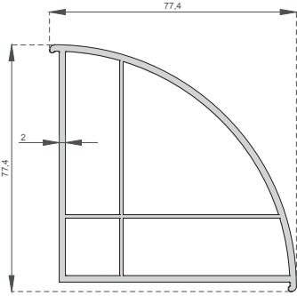
90 Derece Köşe Dönüş Adaptörü 90 Degree Corner Turn Adapter A-1013
