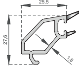
24mm.Cama Göre Çıta Glazing With 24mm.Gap A-1002
