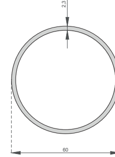
60'lık Boru Profili 60' Pipe Profile A-1014
