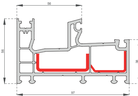
Fix Kasa Profili Fix Frame Profile CS-1006
