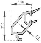
30mm.Cama Göre Çıta Glazing With 30mm.Gap A-1001
