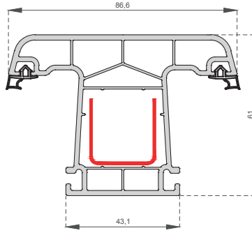
Orta Kayıt Profili Mullion Profile C-6002
