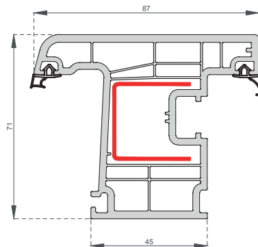
Dışa Açılır Kanat Profili Outward Opening Sash Profile C-7108
